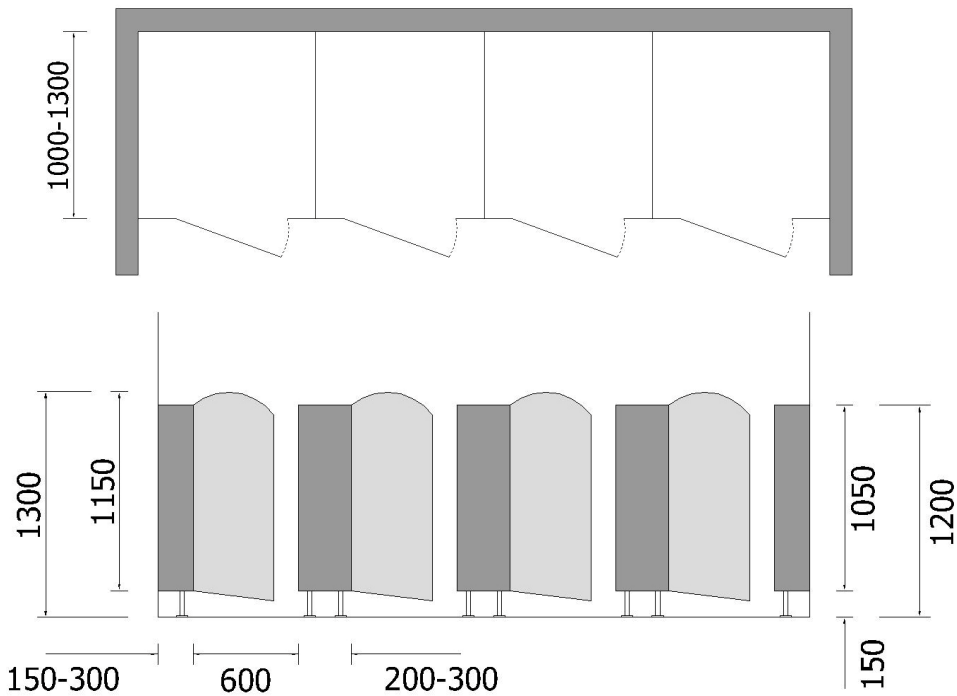
Τυπικές διαστάσεις / Typical dimensions
