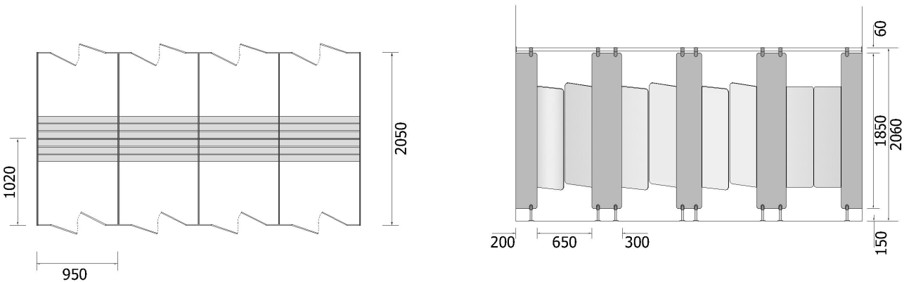
Κεντρικά αποδυτήρια, άνοιγμα πόρτας ale retour / Island version, door opening ale retour
