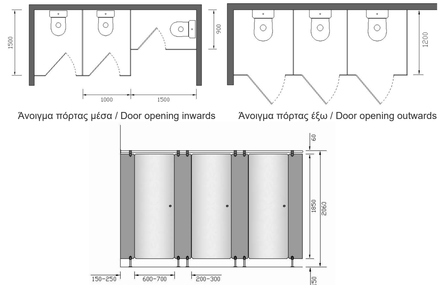
Τυπικές διαστάσεις / Typical dimensions
