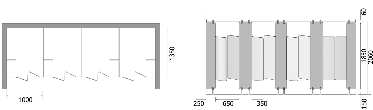
Άνοιγμα πόρτας ale retour / Door opening ale retour
